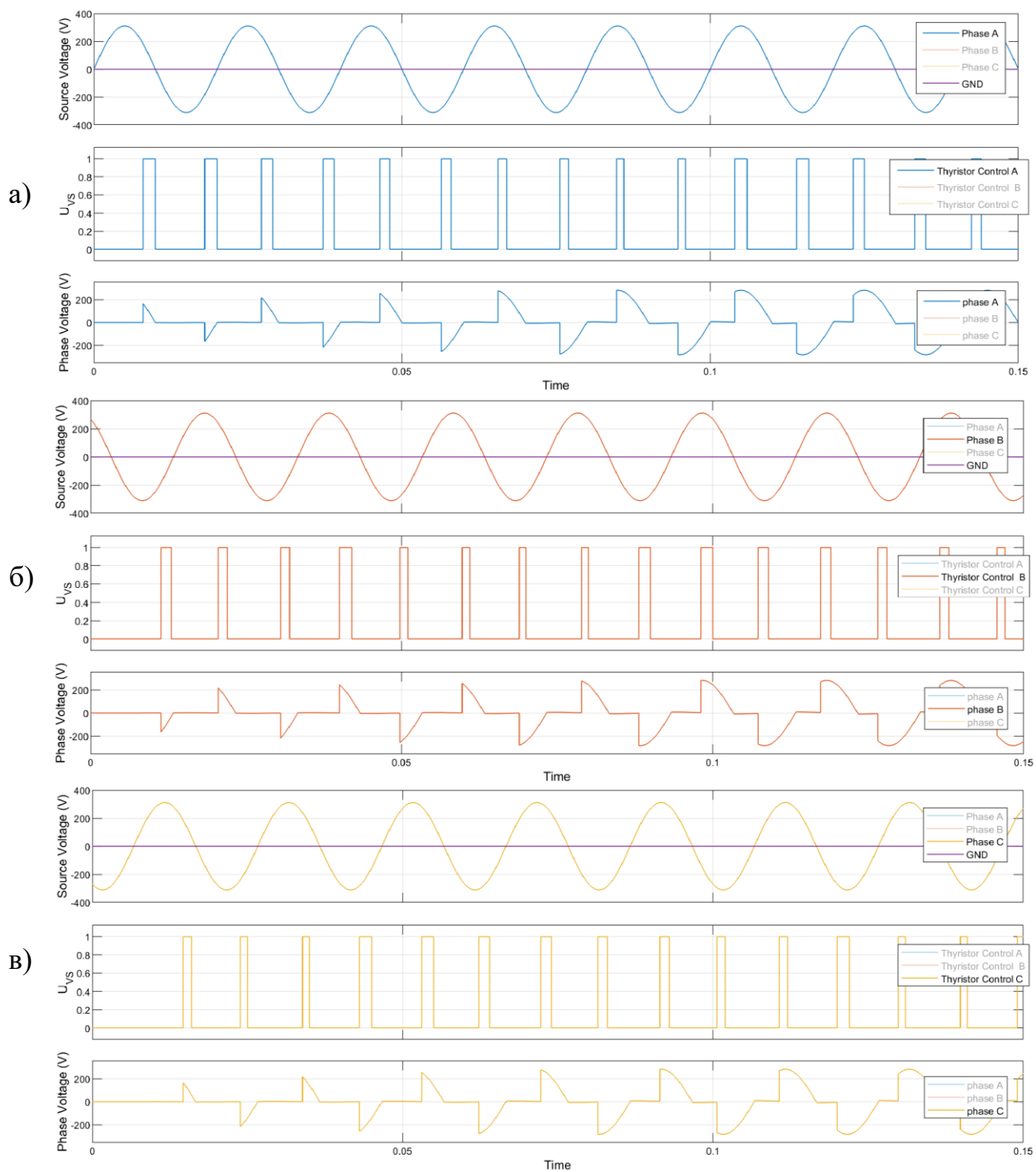
Рисунок 20 – Результаты моделирования исправленного алгоритма определения перехода через ноль
