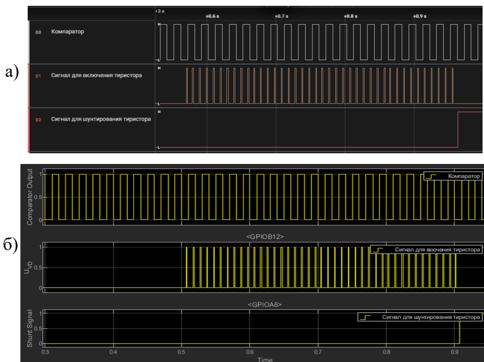
Рисунок 26 – Сравнение модели и реального микроконтроллера
