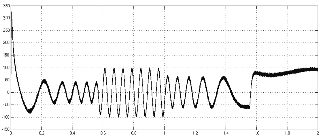
Рис. 9. График тока статора двигателя
