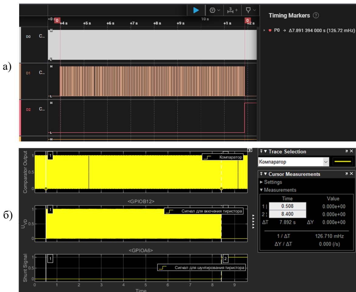
Рисунок 27 – Демонстрация одинакового времени пуска
