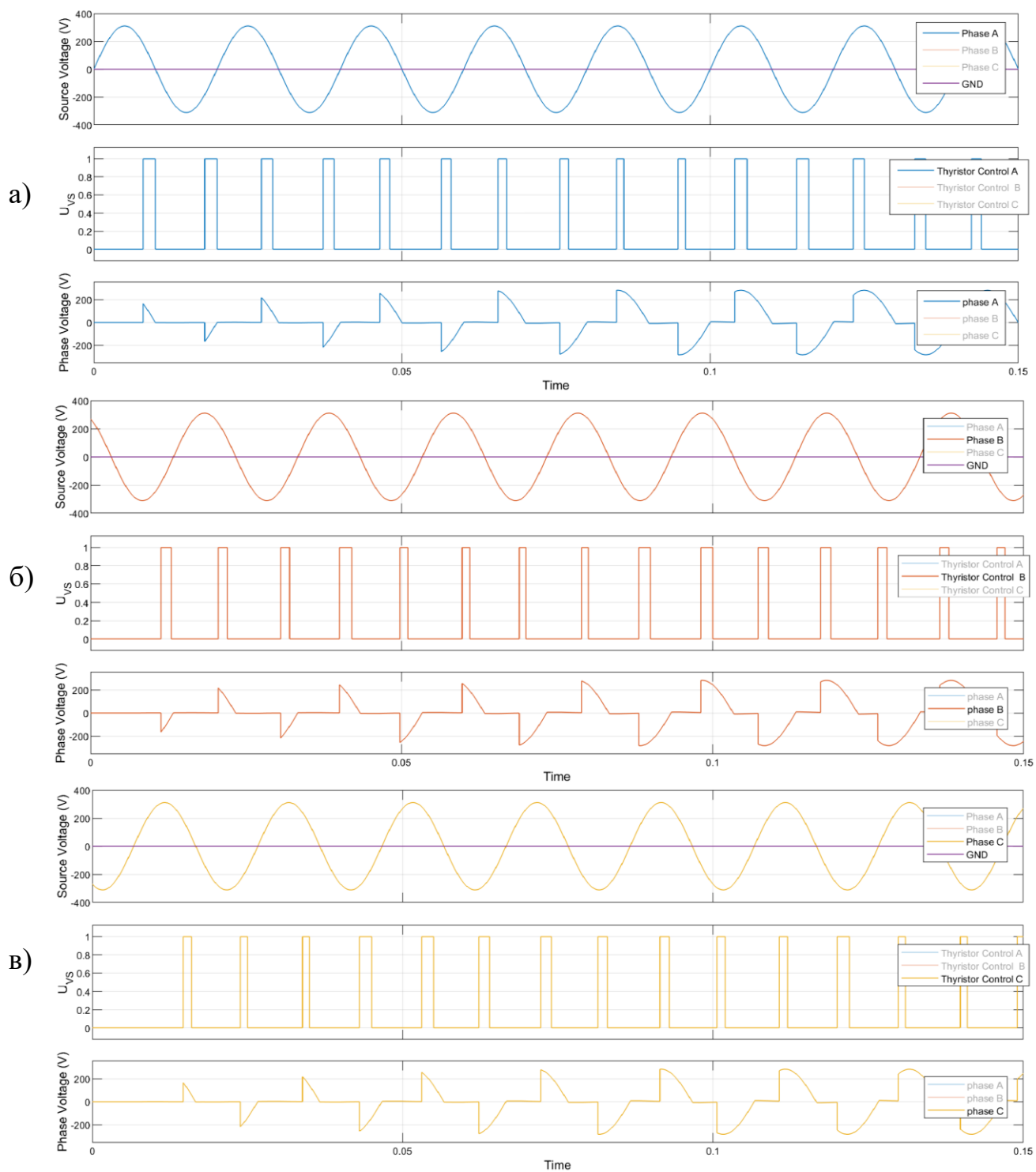
Рисунок 20 – Результаты моделирования исправленного алгоритма
