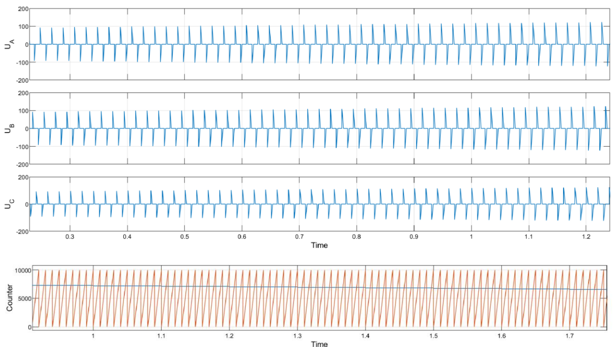
Рисунок 23 – Корректная работа алгоритма расчета угла включения тиристора
