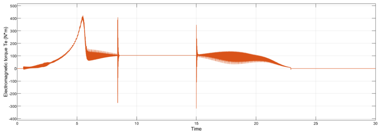
Рисунок 35 – Результаты моделирования прямого пуска асинхронного двигателя
