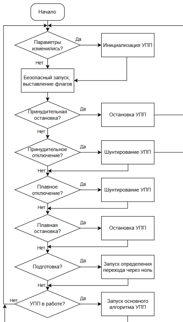
Рисунок 20 – Блок схема управления состоянием УПП
