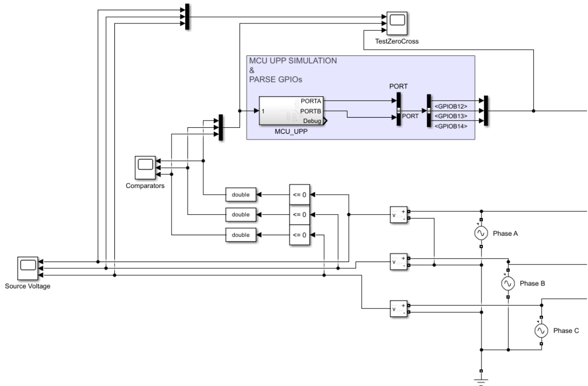
Рисунок 12 – Модель для тестирования алгоритма определения перехода через ноль
