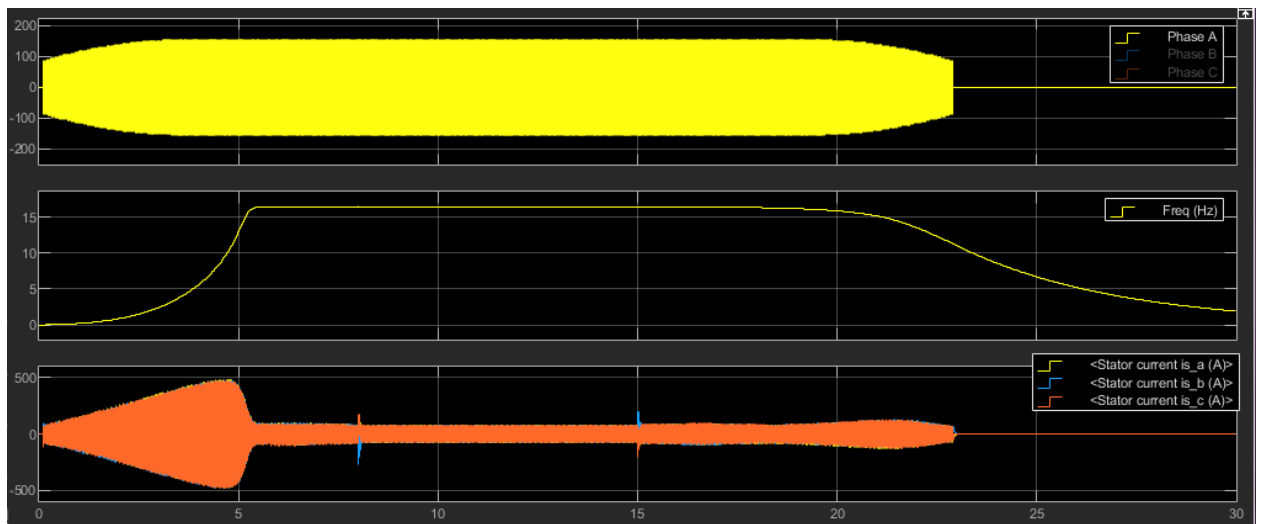
Рисунок 28 – Результаты моделирования прямого пуска асинхронного двигателя
