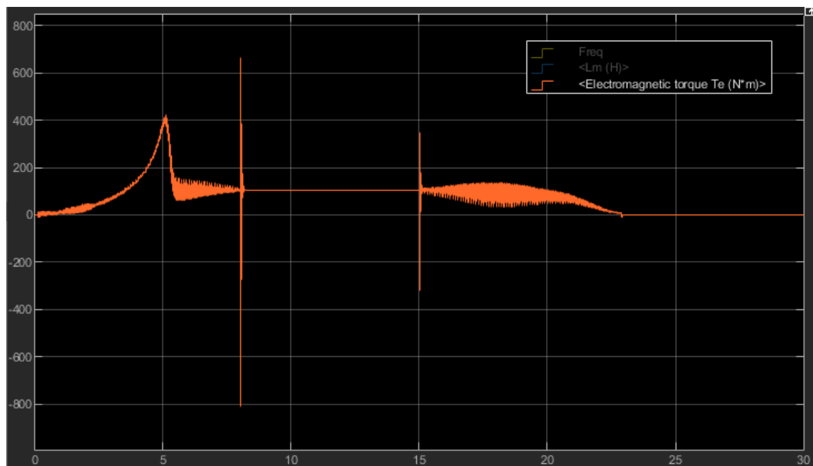
Рисунок 27 – Результаты моделирования прямого пуска асинхронного двигателя
