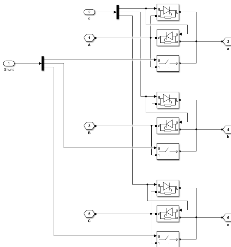
Рисунок 9 – Модель тиристорного модуля
