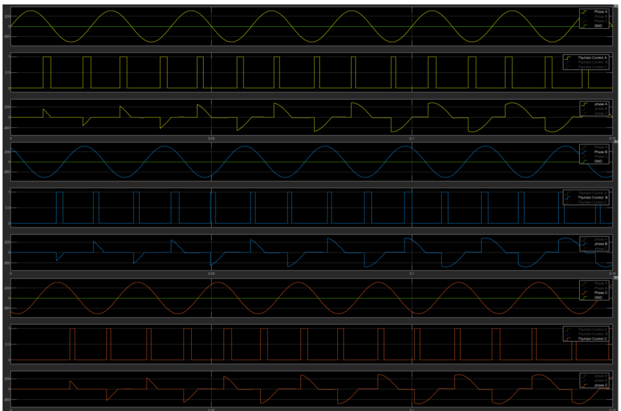
Рисунок 16 – Результаты моделирования исправленного алгоритма определения перехода через ноль
