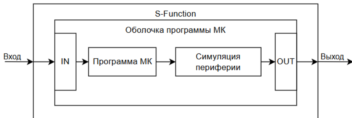
Рисунок 5 – Структурная схема модели микроконтроллера в MATLAB
