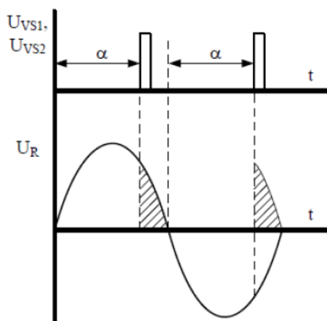
Рисунок 3 – Принцип работы тиристорного регулятора
