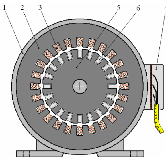
Рисунок 1 – Конструкция асинхронного двигателя
