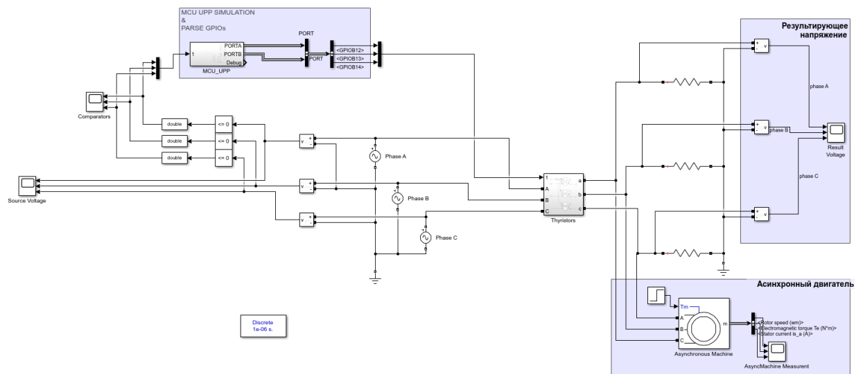
Рисунок 10 – Схема для тестирования алгоритма УПП
