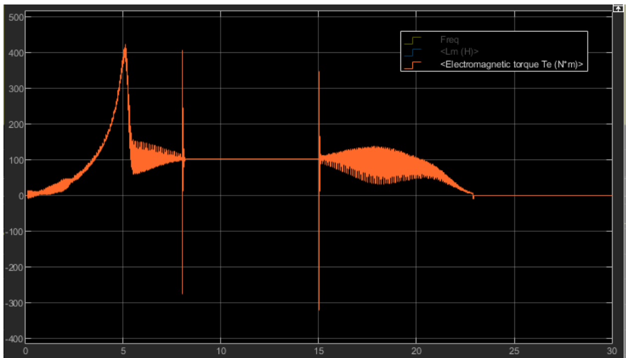
Рисунок 29 – Результаты моделирования прямого пуска асинхронного двигателя
