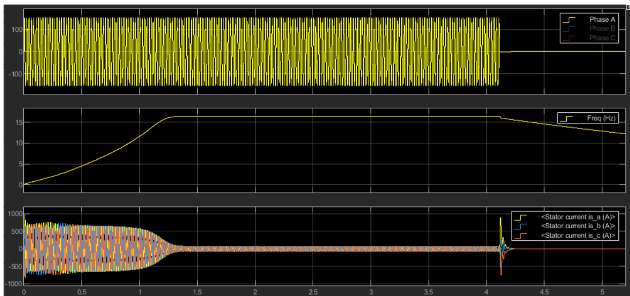
Рисунок 22 – Результаты моделирования прямого пуска асинхронного двигателя
