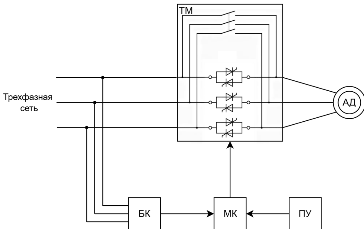
Рисунок 8 – Структурная схема УПП
