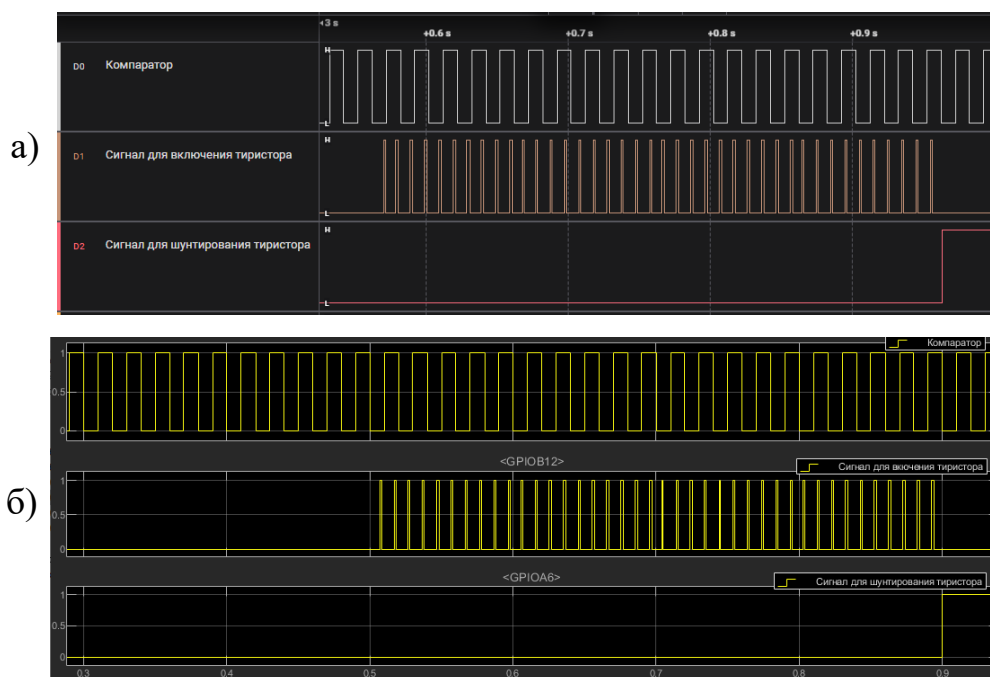
Рисунок 30 – Сравнение модели и реального микроконтроллера
