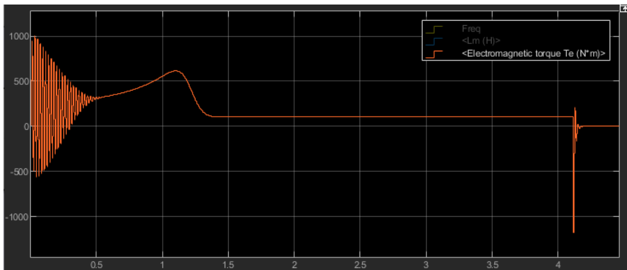
Рисунок 24 – Крутящий момент двигателя при прямом пуске
