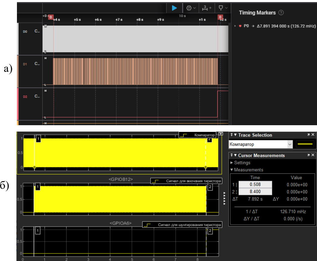
Рисунок 31 – Демонстрация одинакового времени пуска
