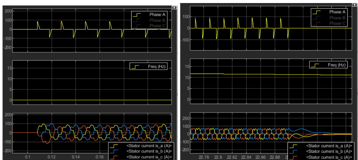
Рисунок 26 – Токи статора асинхронного двигателя в моменты запуска и остановки в режиме плавного пуска
