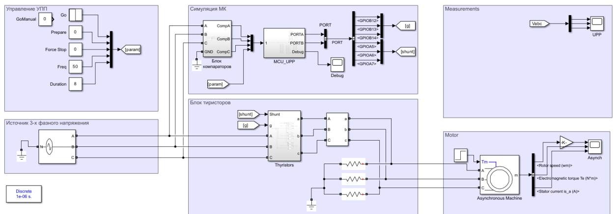
Рисунок 21 – Модель для симуляции УПП
