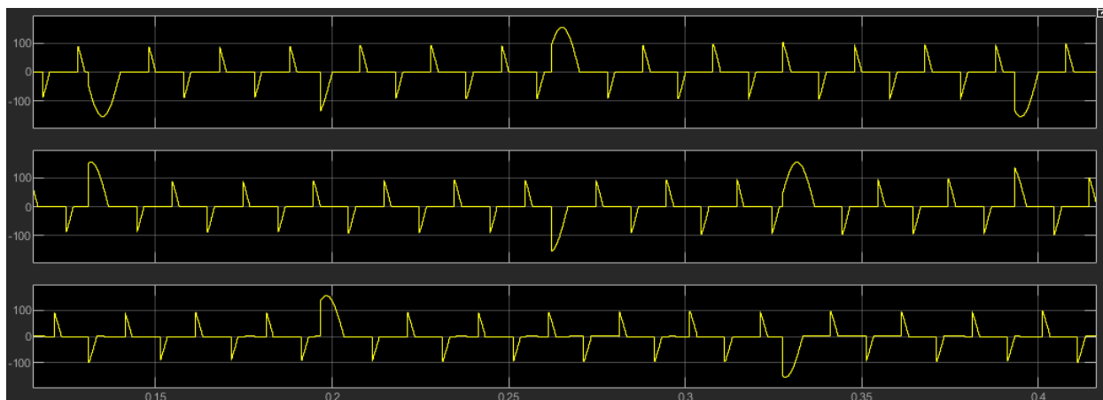
Рисунок 17 – Демонстрация некорректного алгоритма управления тиристорами
