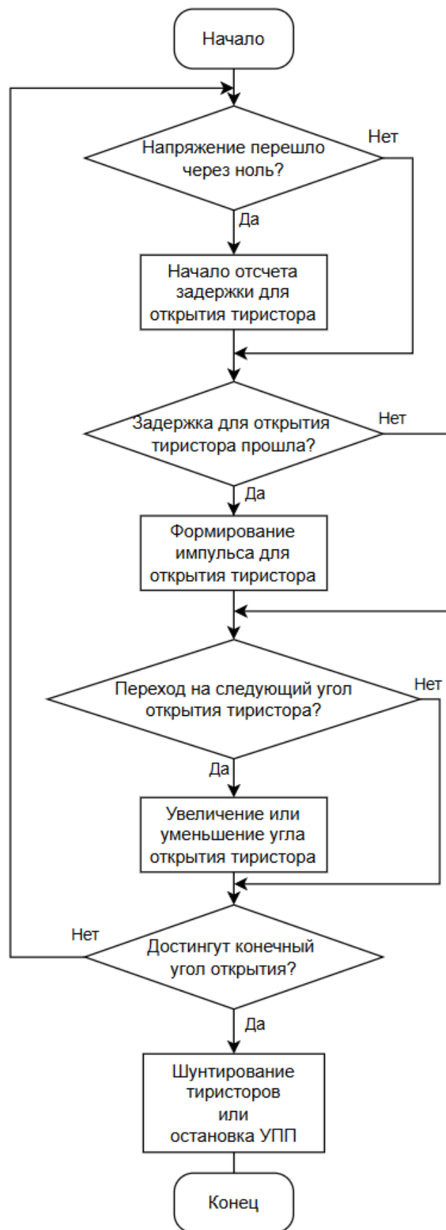
Рисунок 11 – Блок схема алгоритма плавного пуска
