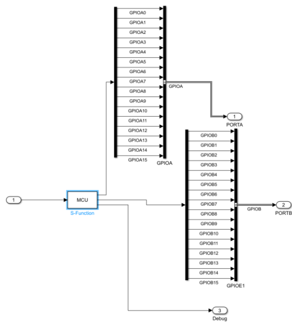
Рисунок 7 – Блок, имитирующий микроконтроллер в MATLAB
