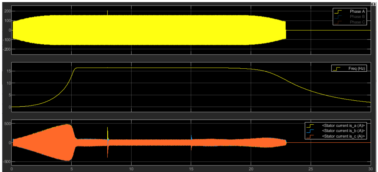
Рисунок 20 – Результаты моделирования пуска асинхронного двигателя через УПП
