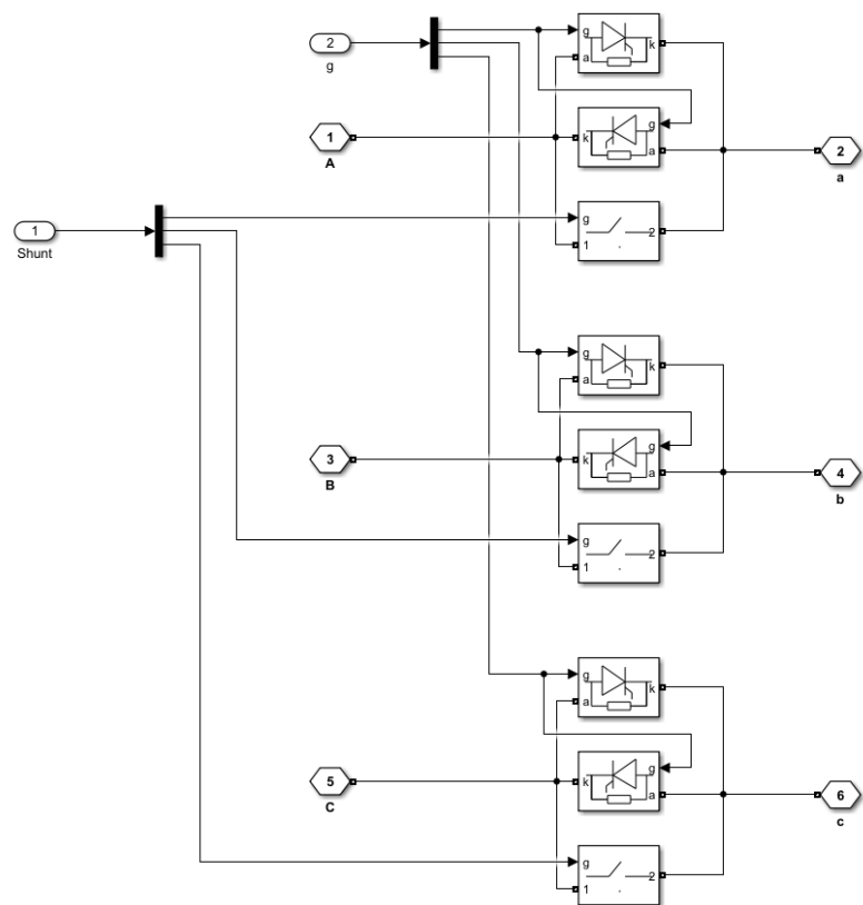
Рисунок 6 – Модель тиристорного модуля
