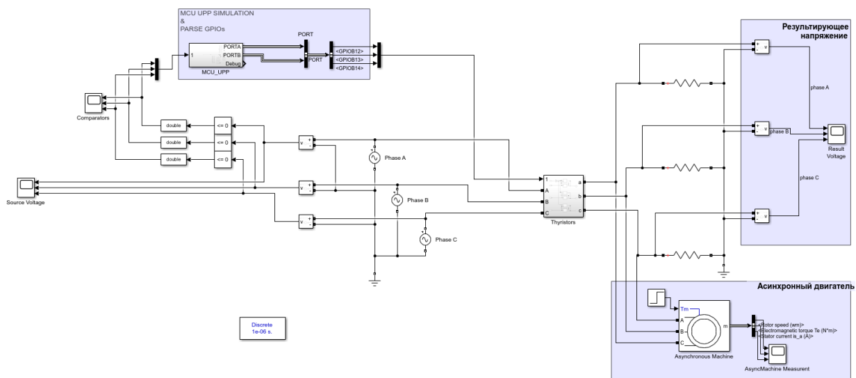
Рисунок 7 – Схема для тестирования алгоритма УПП
