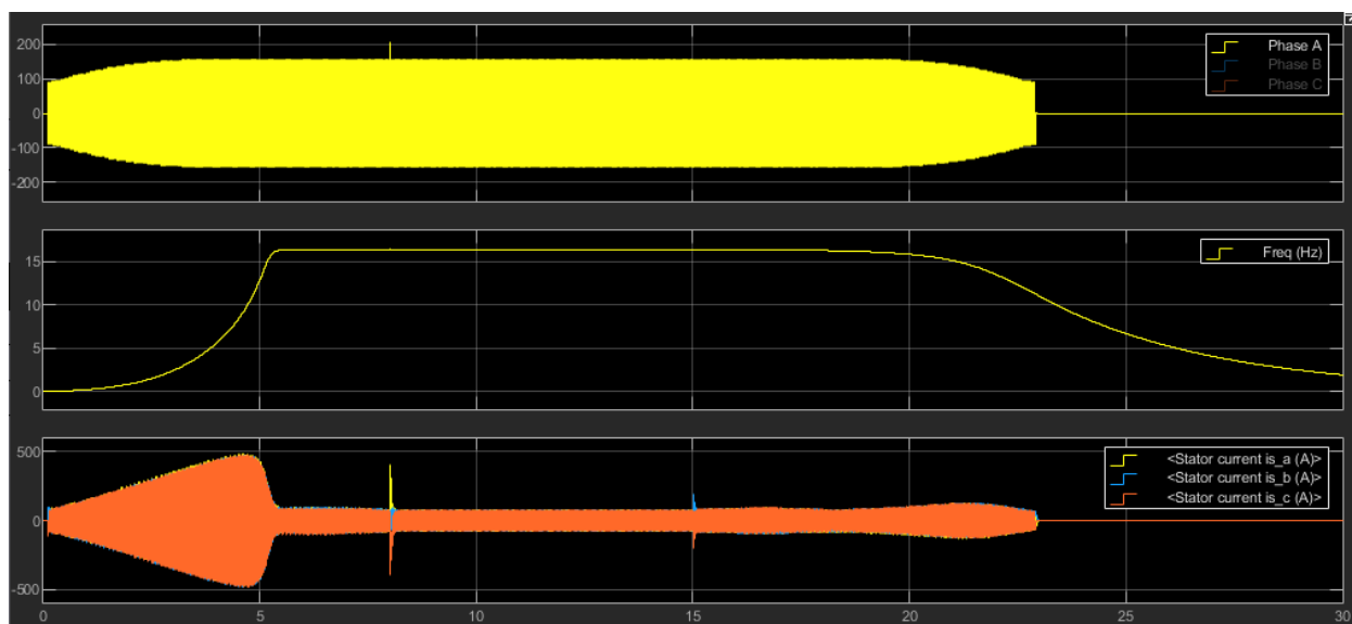
Рисунок 25 – Результаты моделирования пуска асинхронного двигателя через УПП
