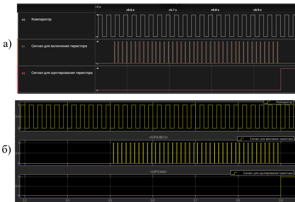
Рисунок 30 – Сравнение модели и реального микроконтроллера
