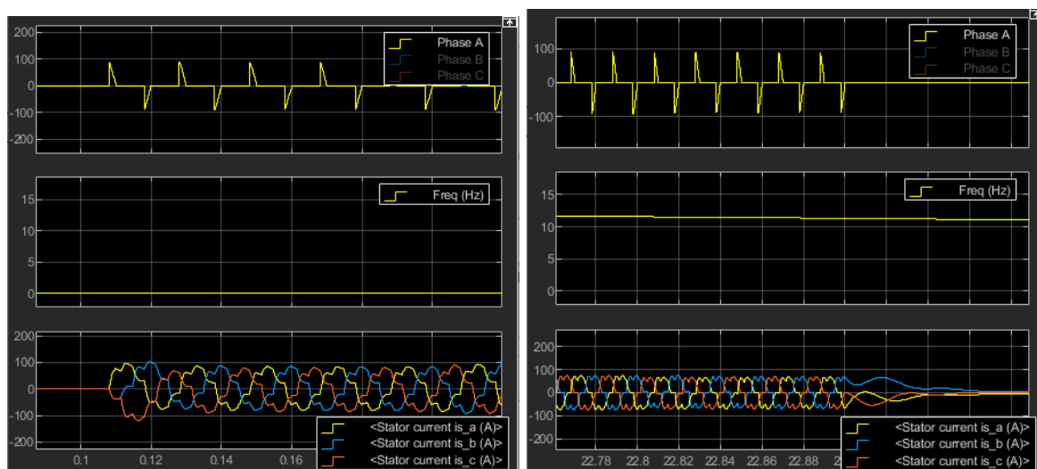
Рисунок 21 – Токи статора асинхронного двигателя в моменты запуска и остановки в режиме плавного пуска
