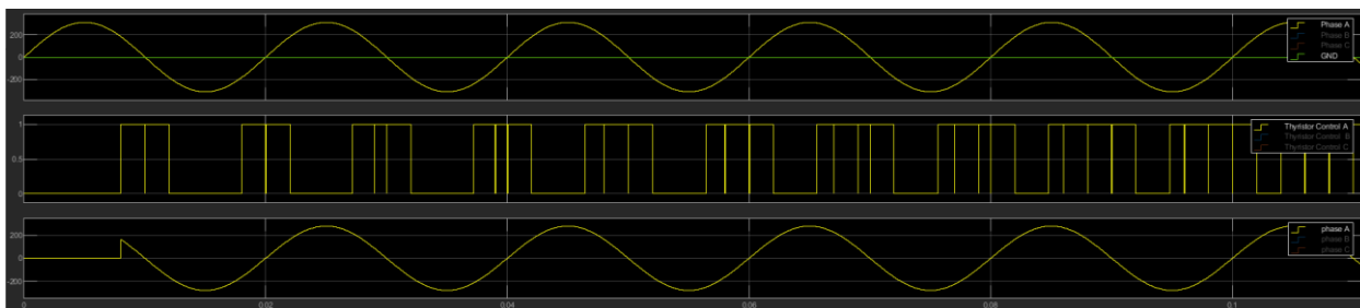
Рисунок 11 – Демонстрация некорректного алгоритма управления тиристорами
