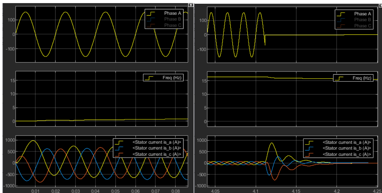
Рисунок 18 – Токи статора асинхронного двигателя в моменты запуска и остановки в режиме прямого пуска
