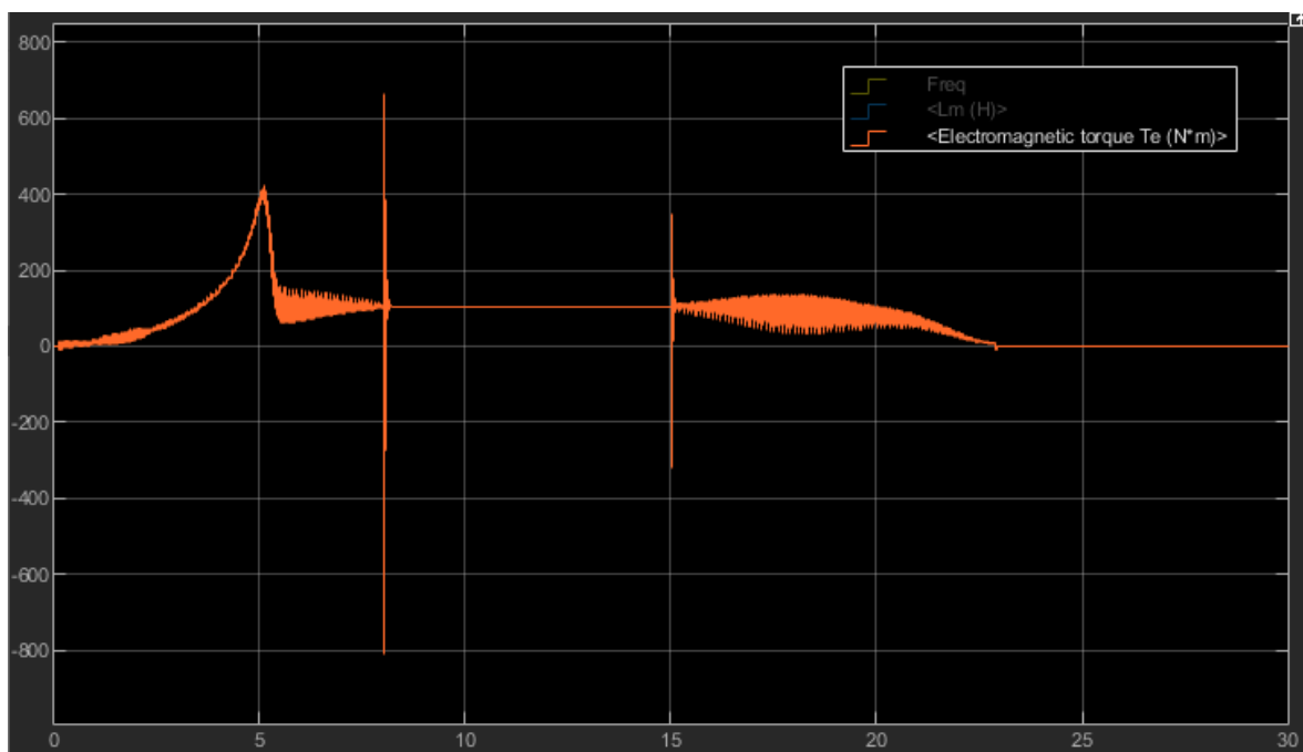
Рисунок 22 – Результаты моделирования прямого пуска асинхронного двигателя
