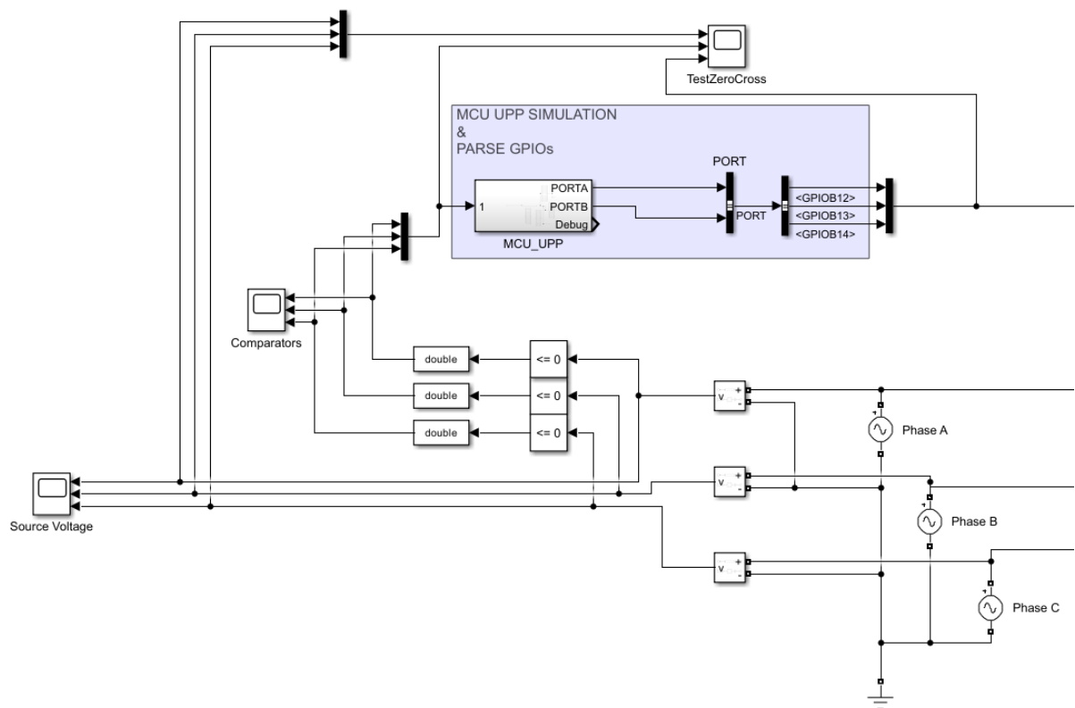
Рисунок 8 – Модель для тестирования алгоритма определения перехода через ноль
