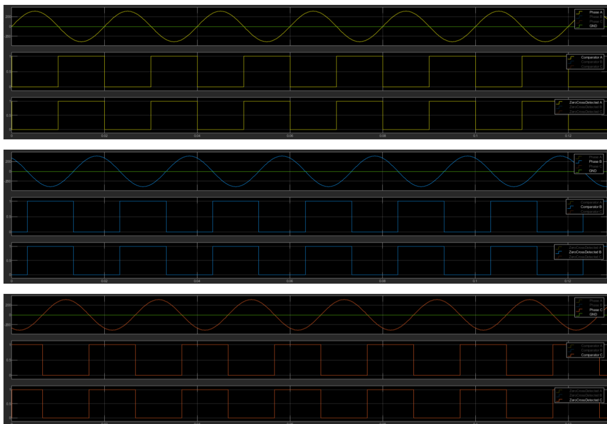
Рисунок 9 – Результаты моделирования алгоритма определения перехода через ноль для каждой фазы
