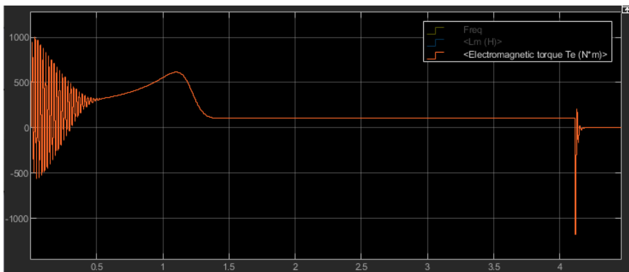
Рисунок 19 – Крутящий момент двигателя при прямом пуске
