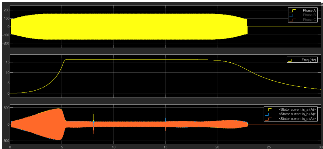
Рисунок 20 – Результаты моделирования пуска асинхронного двигателя через УПП
