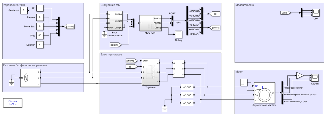
Рисунок 16 – Модель для симуляции УПП
